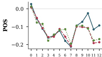
Base GPT-2
